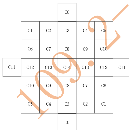
图45 自适应修正滤波系数 (7×7 十字形加 5×5 方形)
