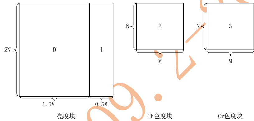
图17 普通帧内编码单元划分为预测块（预测划分方式 ‘VER_RIGHT’）
