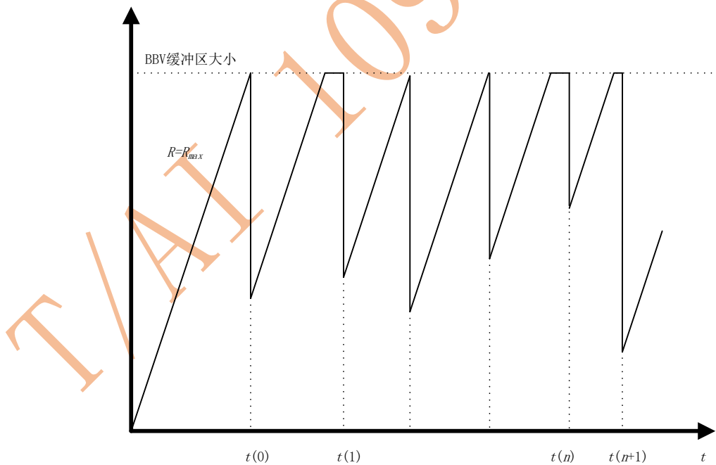
图C.2 BBV 缓冲区占用情况二
