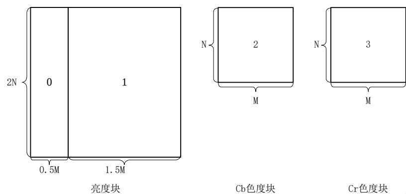
图16 普通帧内编码单元划分为预测块（预测划分方式 ‘VER_LEFT’）
