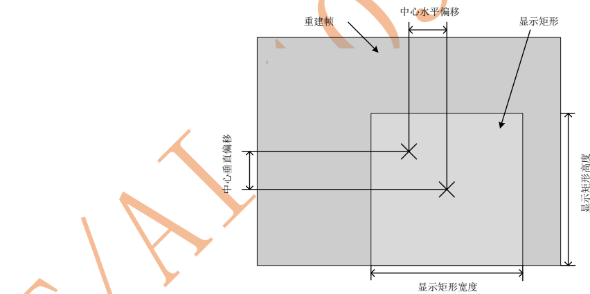
图10 图像中心偏移量参数
