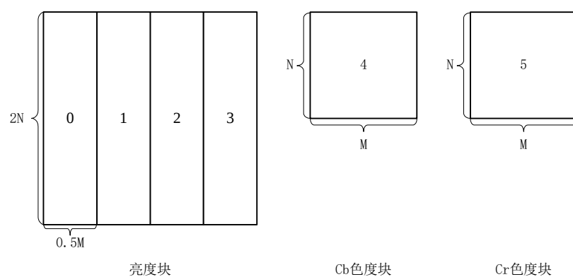
图13 普通帧内编码单元划分为预测块（预测划分方式‘VER_tN’）
