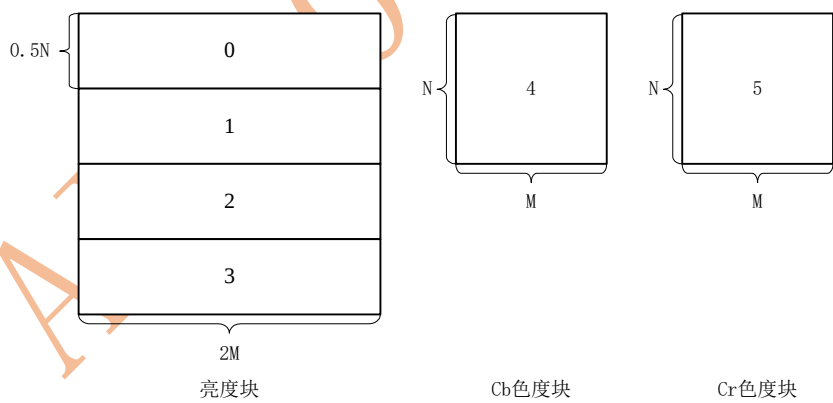
图12 普通帧内编码单元划分为预测块（预测划分方式‘HOR_tN’）
